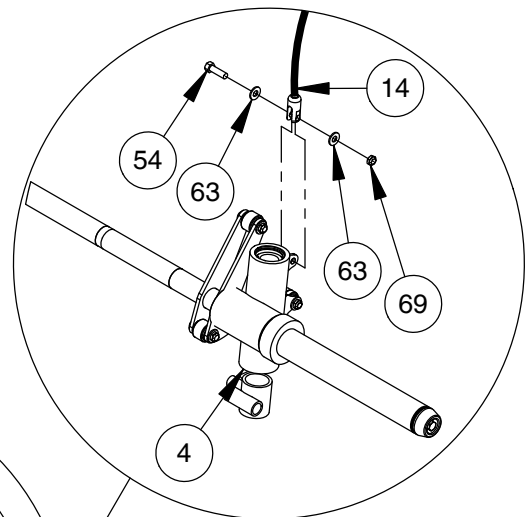
VUE DETAILLE DE L'ANCRAGE DE LA BARRE
