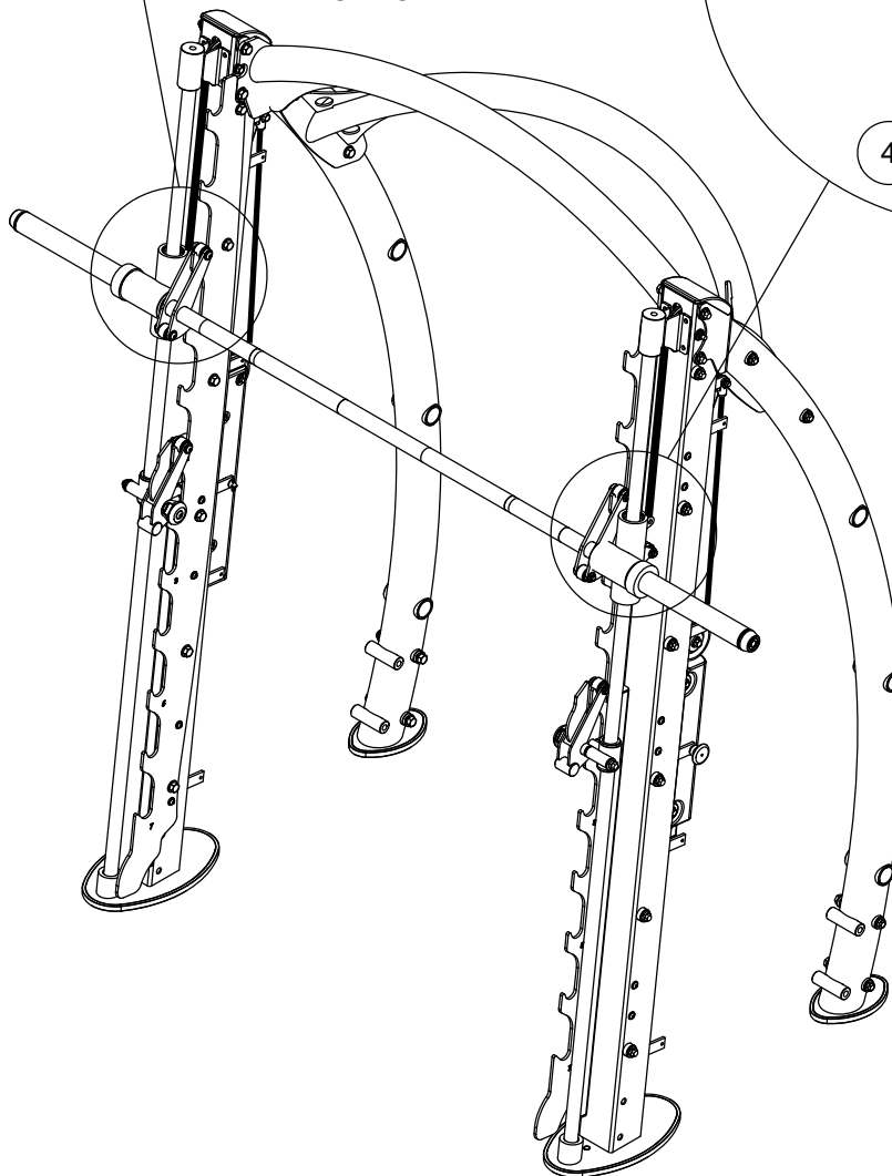
VUE DETAILLE DE L'ANCRAGE DE LA BARRE
